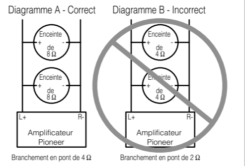
Branchement en pont de 4 Ω Branchement en pont de 2 Ω
